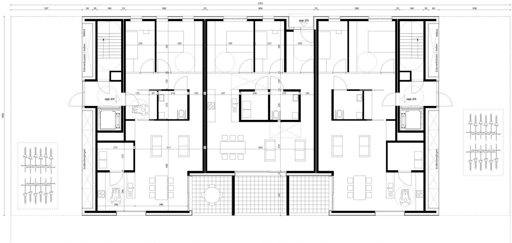
plan gelijkvloers
